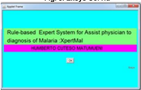
Fig. 3. Exsys Corvid
